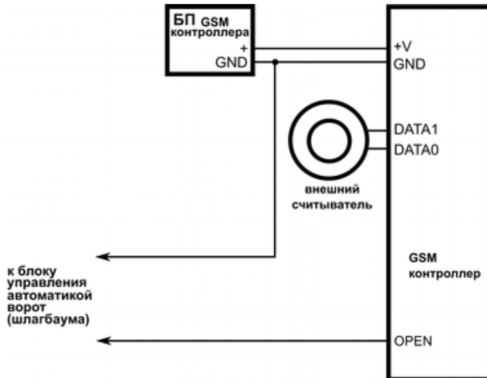
Рис.1 Схема подключения контроллера к блоку управления автоматикой ворот
