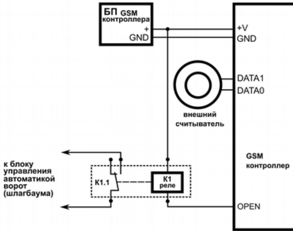
Рис.2 Схема подключения контроллера к блоку управления автоматикой ворот через реле
