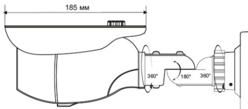
Рис.1 Вид сбоку
