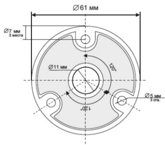
Рис.3 Крепежная платформа
