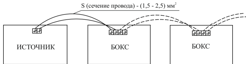
Рисунок 1 – Схема подключения боксов к источнику
